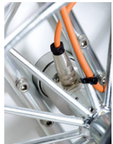
IBAK HSP Schleifringüberträger mit Stecker
