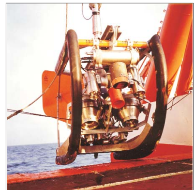
Valdivia Schleppgerät (1972)
