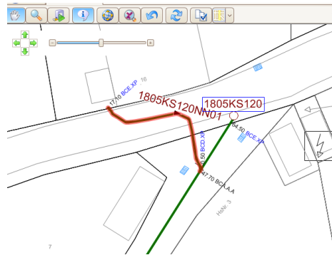
3D-GeoSense-Inspektion mit Live-Rohrverlaufsdarstellung in Plan und Höhenprofil.
