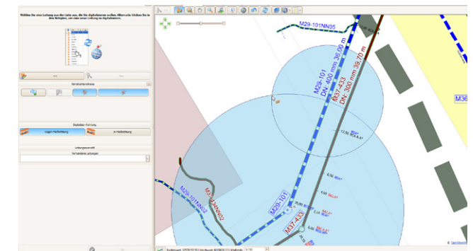
Oben: Live-Verlaufsstellung während der TV-Inspektion Unten: Digitalisierung mit Hilfe von Konstruktionskreisen
