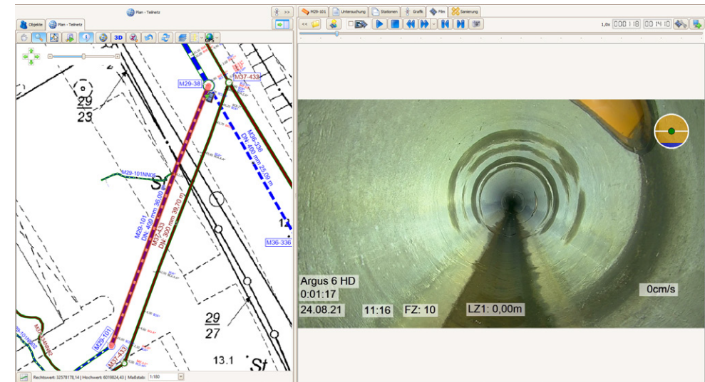
Bearbeitung der Inspektion aus der integrierten GIS-Ansicht
